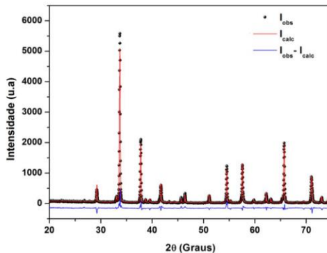
Figura 1. Refinamento de Rietveld para o SrBi 2 Nb 2 O 9 calcinado a 900°C.
