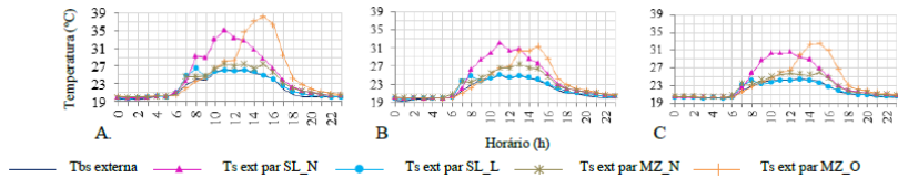
Figura 1. Curvas da Tbs externa e das temperaturas superficiais externa das paredes: para JBCfe (A), Bab_Cab (B), JBCab (C).
