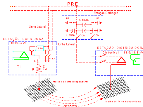
Figura 1. Esquema ilustrativo da tecnologia PRE no esquema trifásico.
