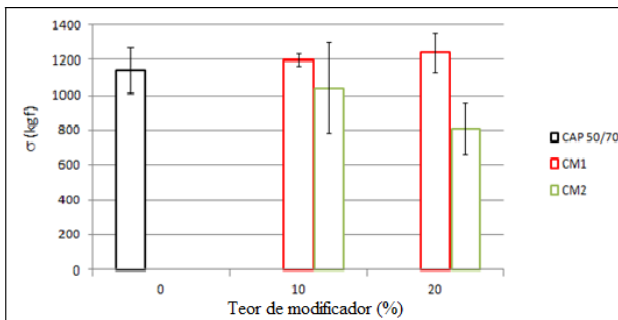
Figura 4. Comportamento da RTCD das misturas em função dos teores de agentes modificadores.
