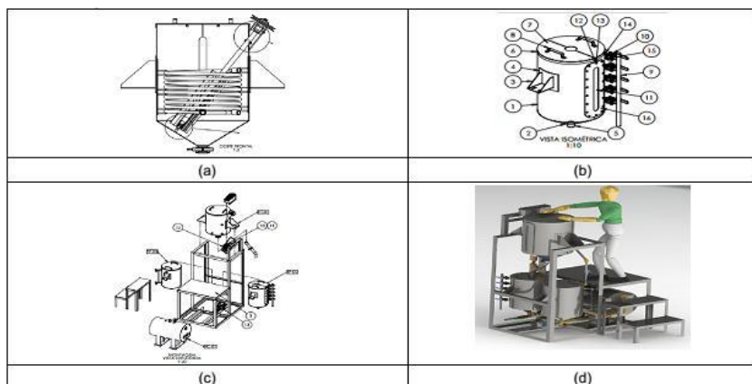
Figura 2. Unidade de extração de óleo – Vista 3D. (a) Reator extrator, (b) tanques de separação de fases, (c) Vista frontal da montagem de cada um dos equipamentos, (d) Unidade montada da unidade extratora.
