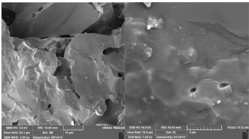
Figura 1. Micrografia do quartzito rosa sinterizados a (a) 1150°C e (b) 1200°C.
