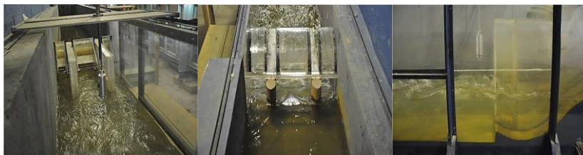
Figura 1. Vista de jusante (esq.), vista de montante (centro) e vista lateral (direita).
