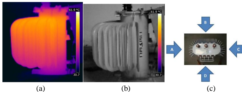
Figura 1. Imagem termográfica da face A do transformador (a), imagem real do transformador (b) e indicações do posicionamento das faces (c).
