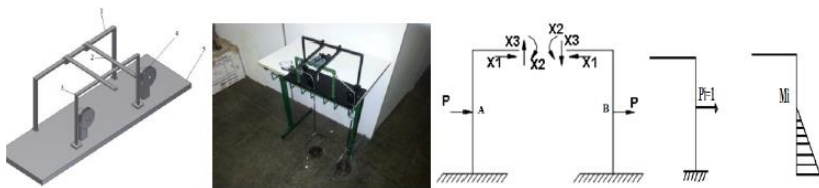
Figura 3. Equipamento fabricado para ensaio de Pórtico hiperestático para determinação dos deslocamentos e diagrama de esforços, momentos reais e unitários, respectivamente.
