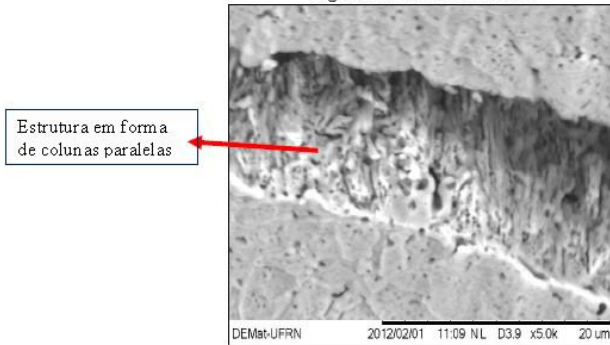
Figura 3 : MEV aumento de 5.000X tratamento térmico a 1700 °C trinca feita para mostrar a região interna de membrana.
