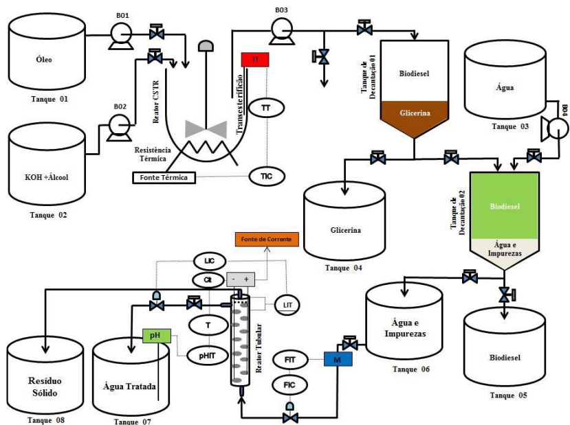
Figura 2. Planta de produção do biodiesel.
