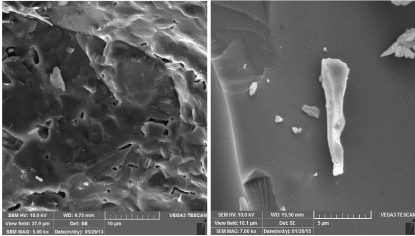
Figura 3. Micrografia do quartzito verde sinterizado a (a) 1150°C e (b) 1200°C.
