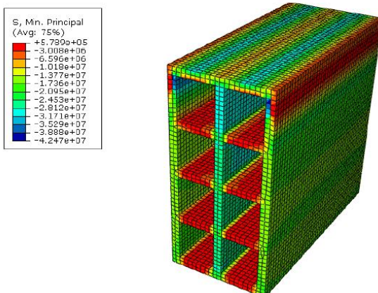
Figura 3. Distribuição de tensões devido à compressão no modelo analisado.
