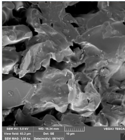
Figura 4. Micrografia do quartzito preto sinterizado a (a) 1150°C.
