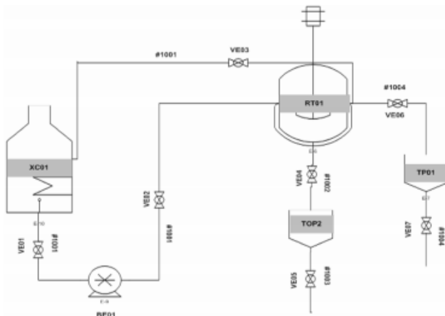
Figura 1. Fluxograma de processo – Unidade de extração de óleo.
