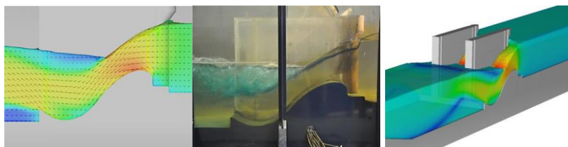
Figura 4. Padrão do escoamento Flow3D (esquerda e direita) e modelo experimental (centro).
