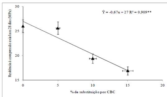
Figura 3. Resultados do ensaio de resistência à compressão axial aos 28 dias em função da substituição de cimento Portland por CBC. ** significativo ( P < 0,01 ).
