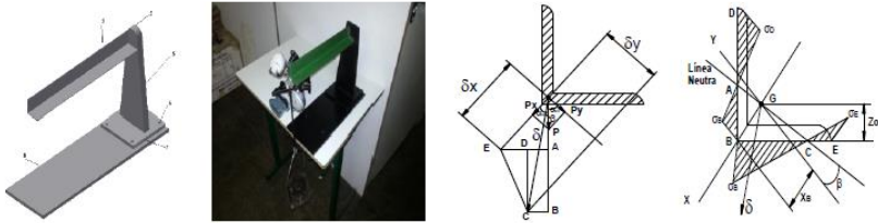
Figura 2. Equipamento fabricado para ensaio de Flexão Oblíqua e diagrama de esforços e distribuição de tensões normais, respectivamente.
