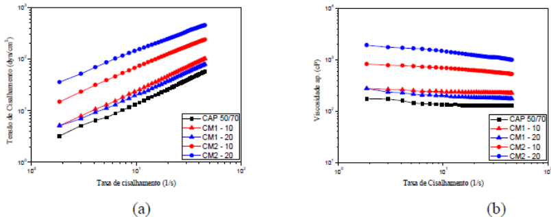
Figura 3: Comportamento reológico em regime permanente do CAP 50/70 e ligantes modificados - CM1-10; CM1-20; CM2-10 e CM2-20, na temperatura de 170°C: (a) tensão cisalhamento versus taxa de cisalhamento e (b) viscosidade aparente versus taxa de cisalhamento.
