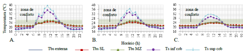
Figura 3. Curvas das temperaturas do ar exterior, na sala e no mezanino e das temperaturas superficiais da cobertura: para JBCfe (A), Bab_Cab (B) JBCab (C).
