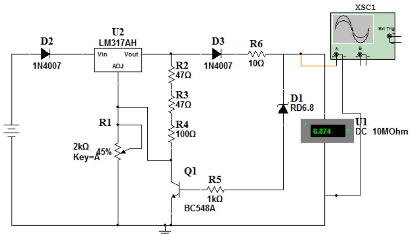
Figura 1. Circuito do carregador em ambiente virtual.
